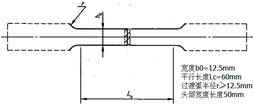
图 1 铝型材拉伸试样图示
