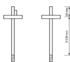
图 4 抗剪力试验试样示意图
