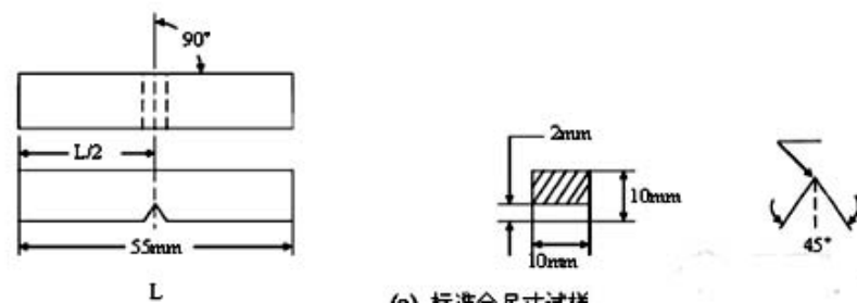
图6 钢材冲击试验（左边 V 型缺口，右边 U 型缺口）
